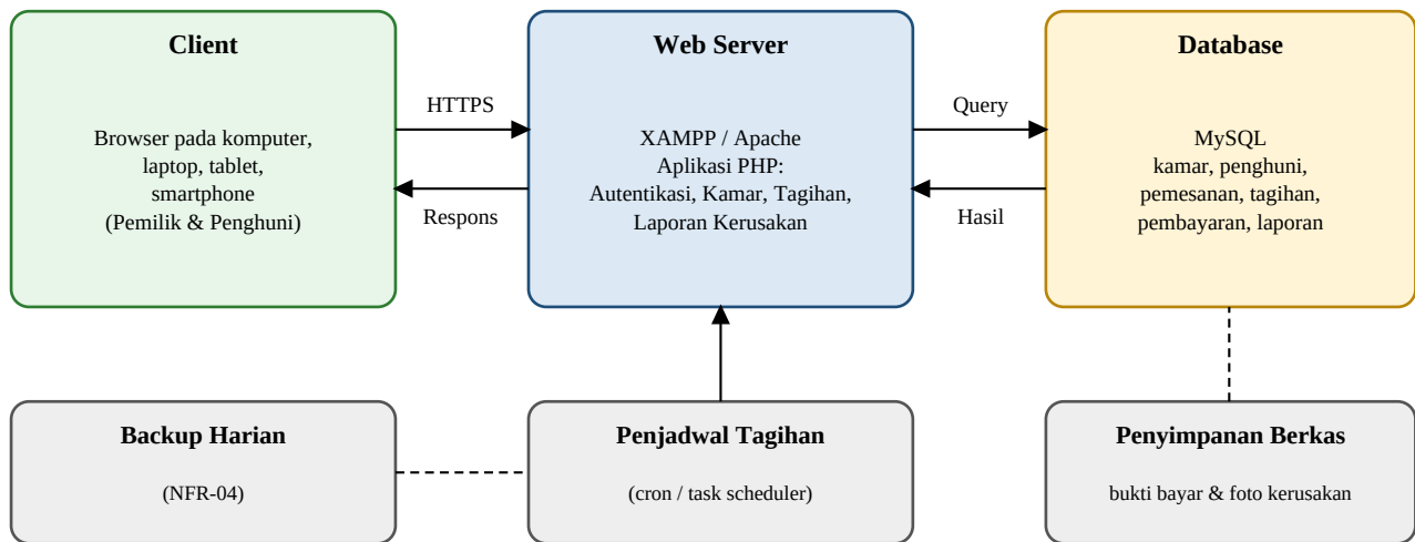
Gambar D.6 Arsitektur Sistem Informasi Manajemen Kos-Kosan
