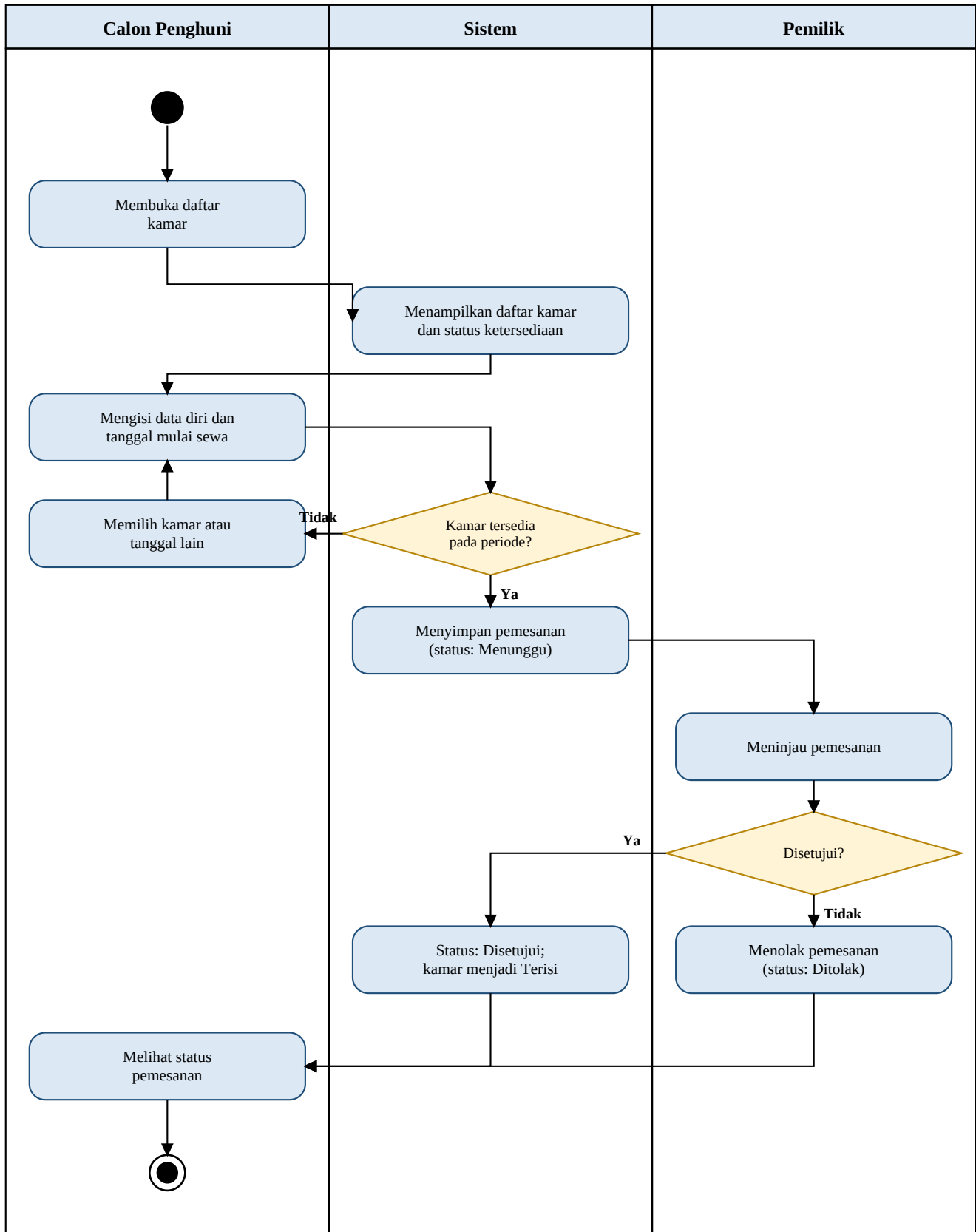
Gambar D.2 Activity Diagram Pemesanan Kamar
