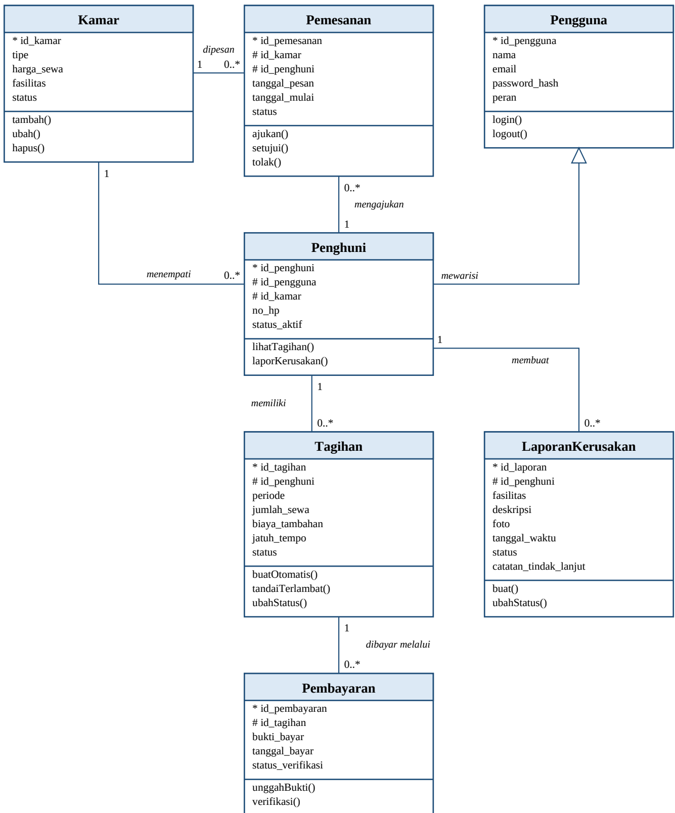
Gambar D.5 Class Diagram Sistem Informasi Manajemen Kos-Kosan
